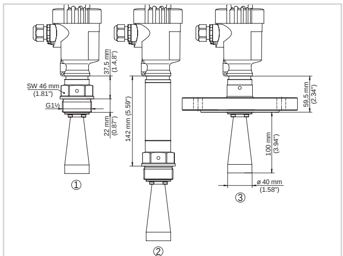
Dimensions VEGAPULS 62
