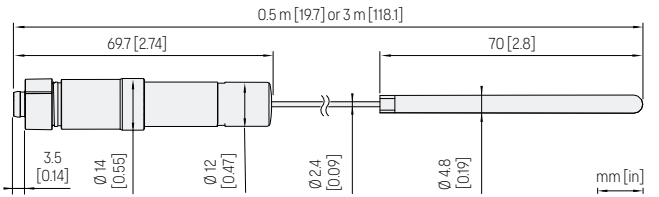
TMP115 dimensions
